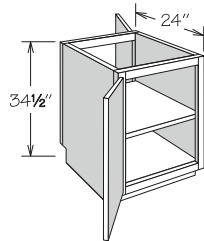
2 DOORS
