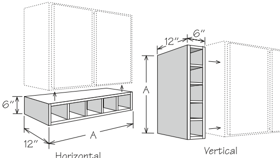
30" Shown
